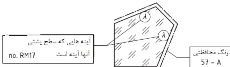
شکل ۱ - مثالی از نمایش عملیات سطح محافظتی (قطر خارجی mm(48 \pm 0,05) مربوط به قطعه بعد از رنگ‌کاری است)
