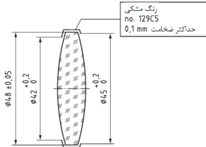
شکل ۱ - مثالی از نمایش عملیات سطح محافظتی (قطر خارجی mm(48 \pm 0,05) مربوط به قطعه بعد از رنگ‌کاری است)
