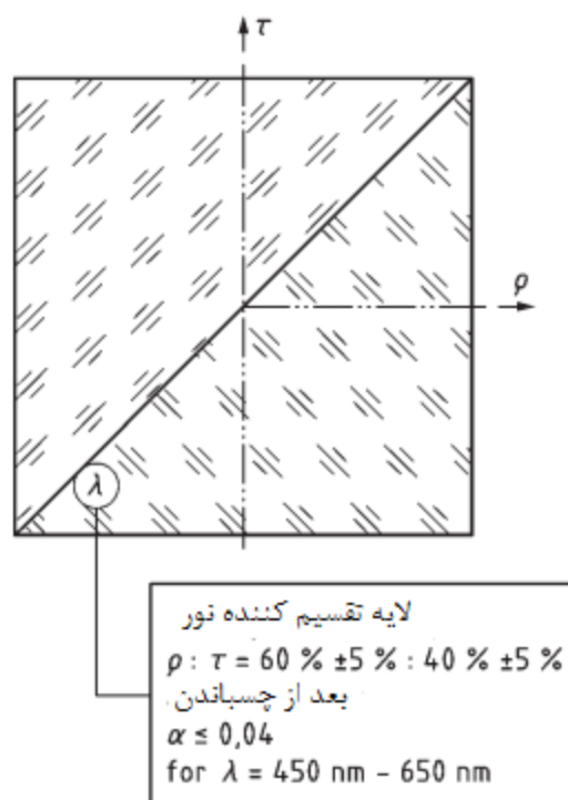
شکل ۳- مثالی از نمایش لایه نشانی کارکردی با ویژگی های نهادهای اپتیکی
