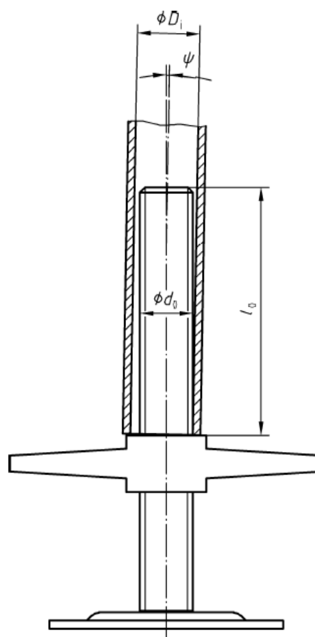
شکل ۸ - زاویه‌ی انحراف بین یک پایه و یک پایه‌ی لوله‌ای
