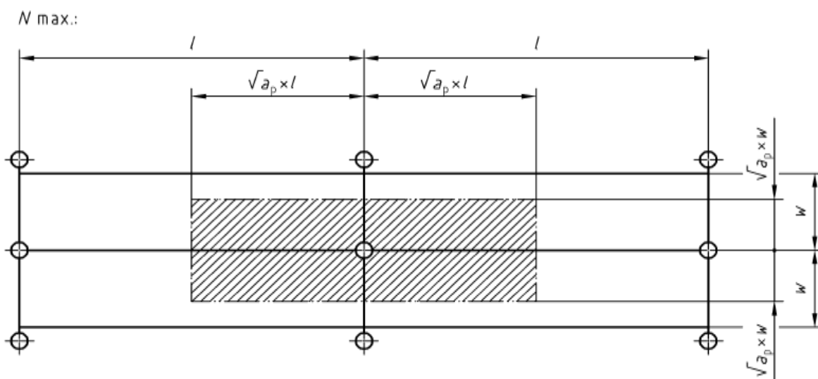
د- پایه‌ی مرکزی داربست قفسه بندی (مشبک)
