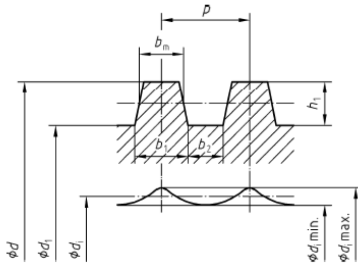
شکل ب-۲ - رزوه دوزنقه‌ای
