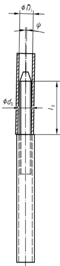
شکل ۷ - زاویه انحراف بین پایه‌های لوله‌ای
